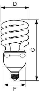
EcoHL Twist 45W CDL E27 220-240V 50/60Hz
